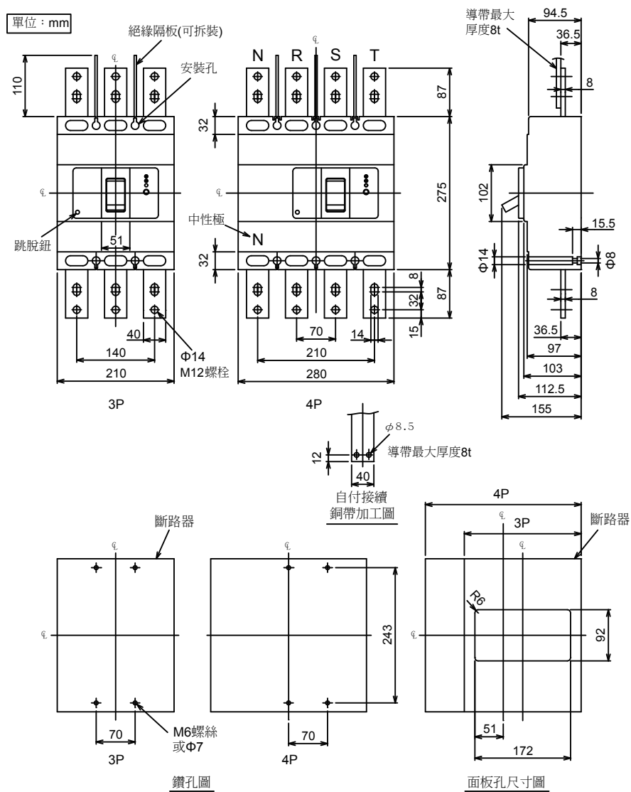
NV800-RN 3P/4P(500A,600A,630A) 外型尺寸圖
