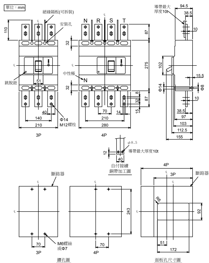
NV800-RN 3P/4P( 700A,800A) 外型尺寸圖
