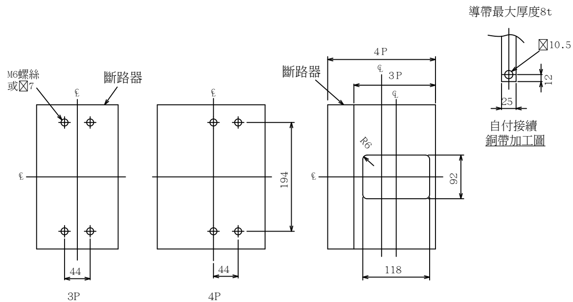
鑽孔圖
