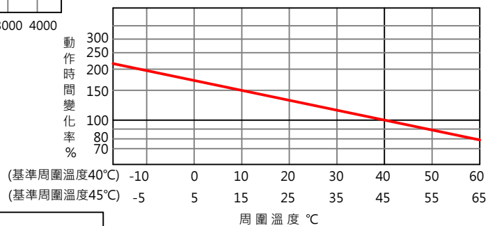
溫度特性曲線
