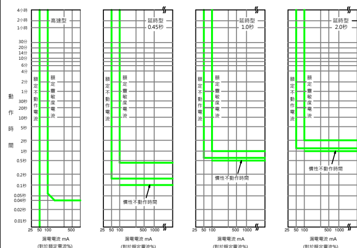
漏電跳脫特性曲線
