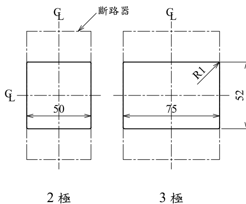
面板孔尺寸圖
