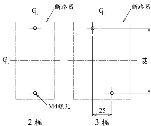
鑽孔圖
