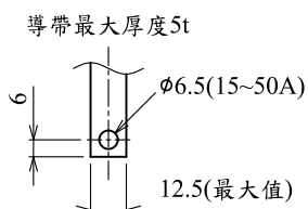
自付接續 銅帶加工圖
