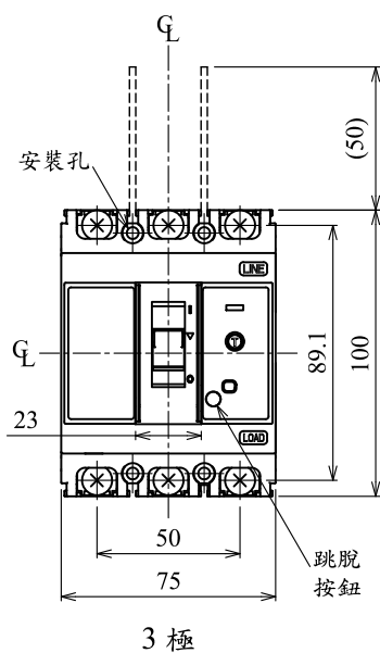
外型尺寸圖
