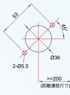
門板鑽孔圖
