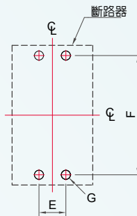
斷路器鑽孔圖
